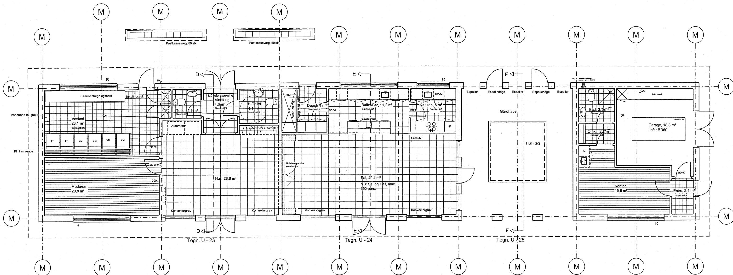
PLAN FÆLLESHUS, 1 : 100
